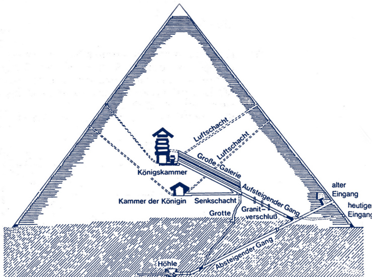
De inhoud van de piramide van Chephren
